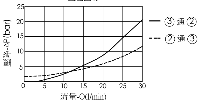
性能曲線
