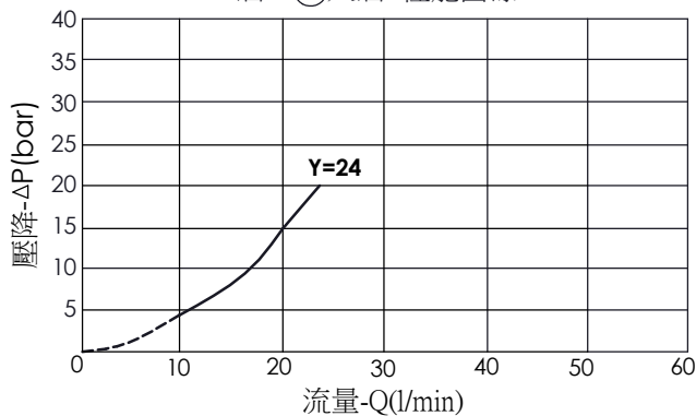
油口③入油 性能曲線
