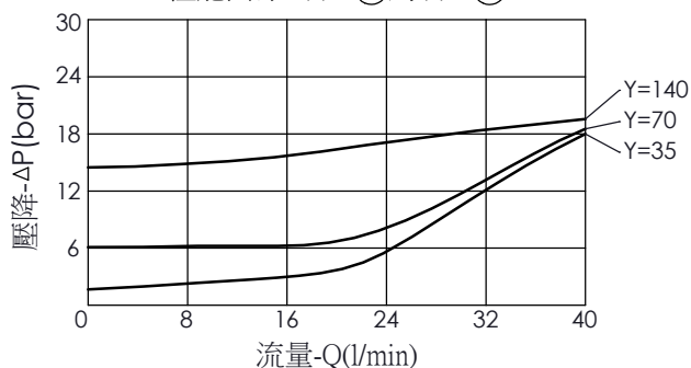
性能曲線 油口①到油口②
