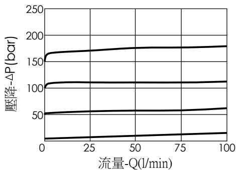
洩壓曲線
