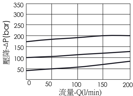
洩壓曲線
