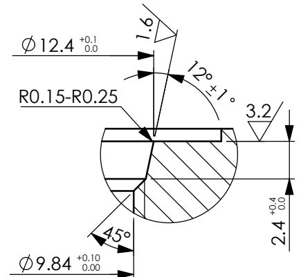
細部放大圖 C
