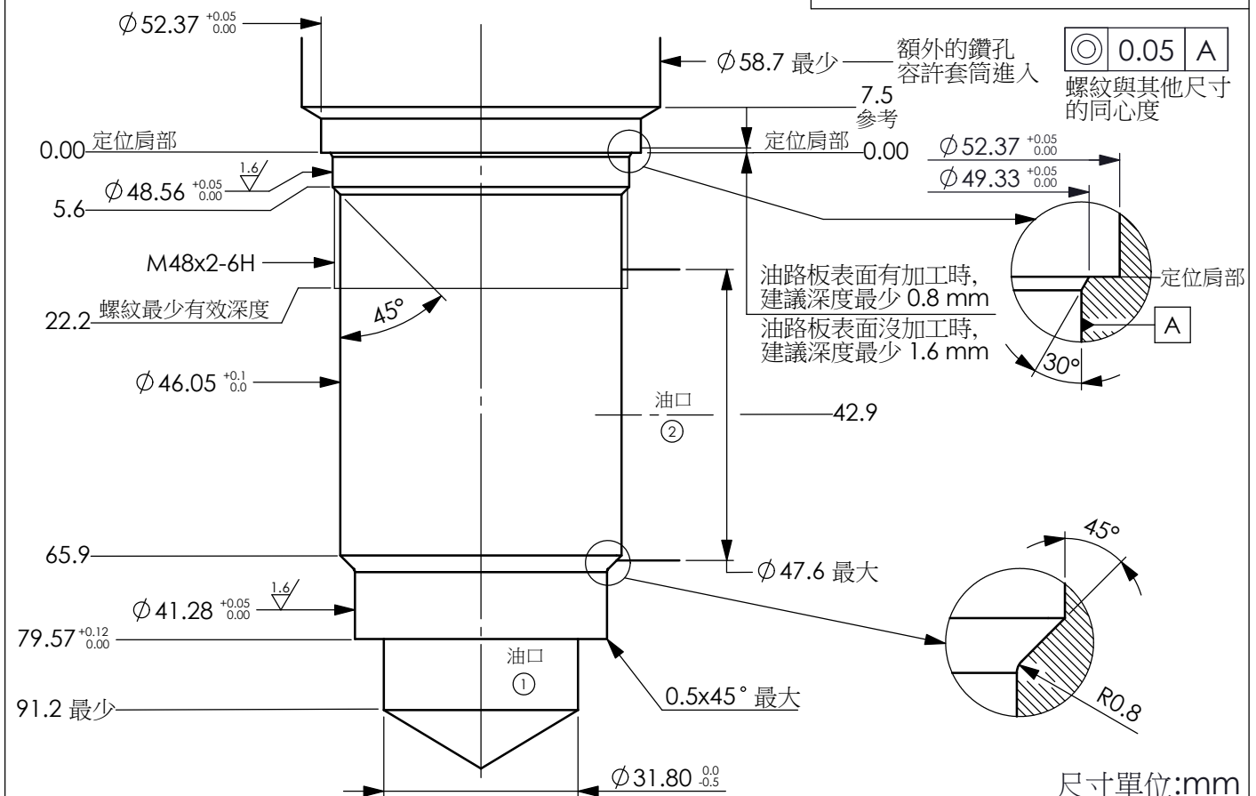
成型孔:18A-2
