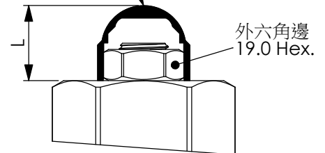
H19螺帽塑膠保護蓋
